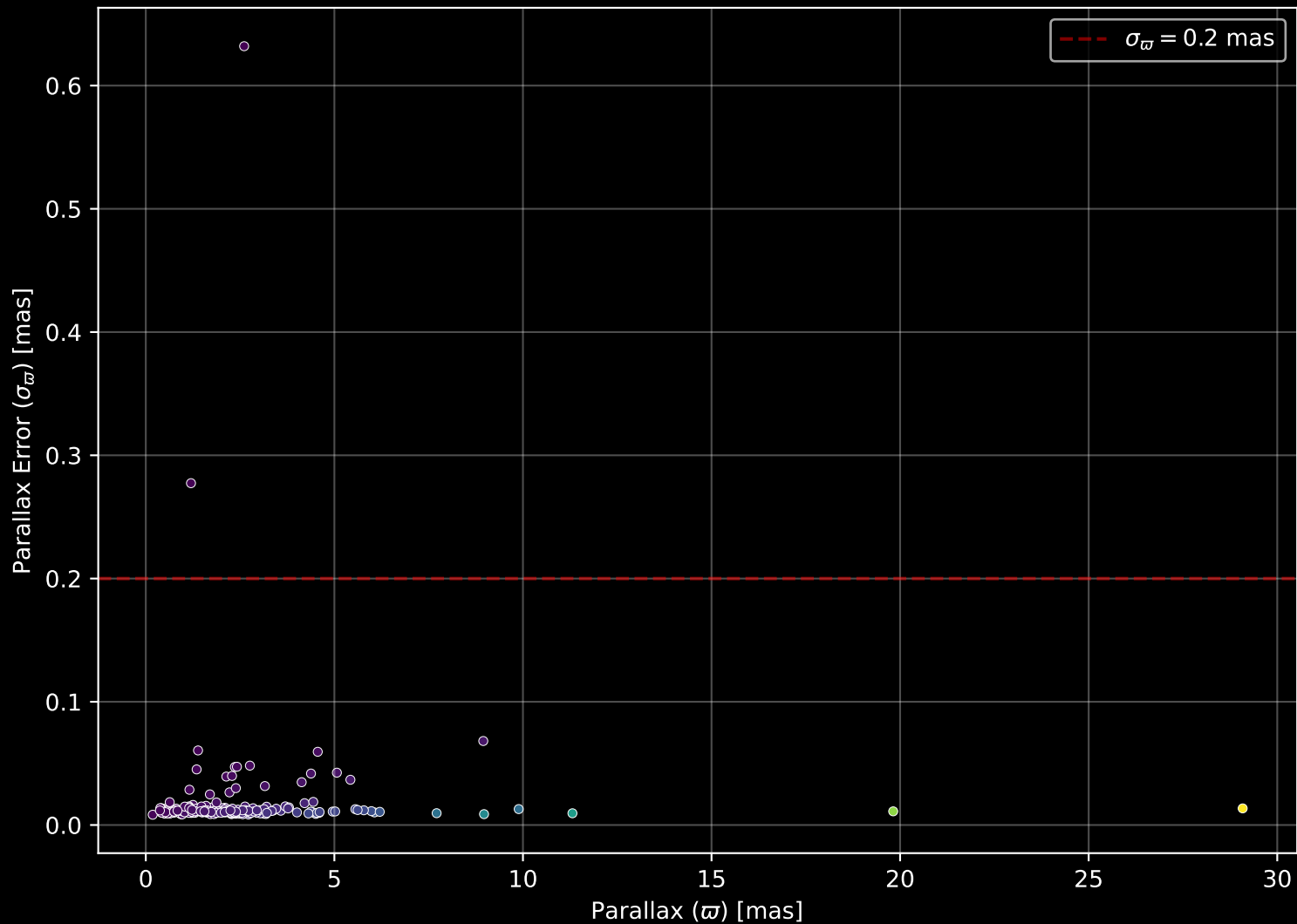
GALAH DR4 Field: [7238] Parallax Quality (n= 209)
