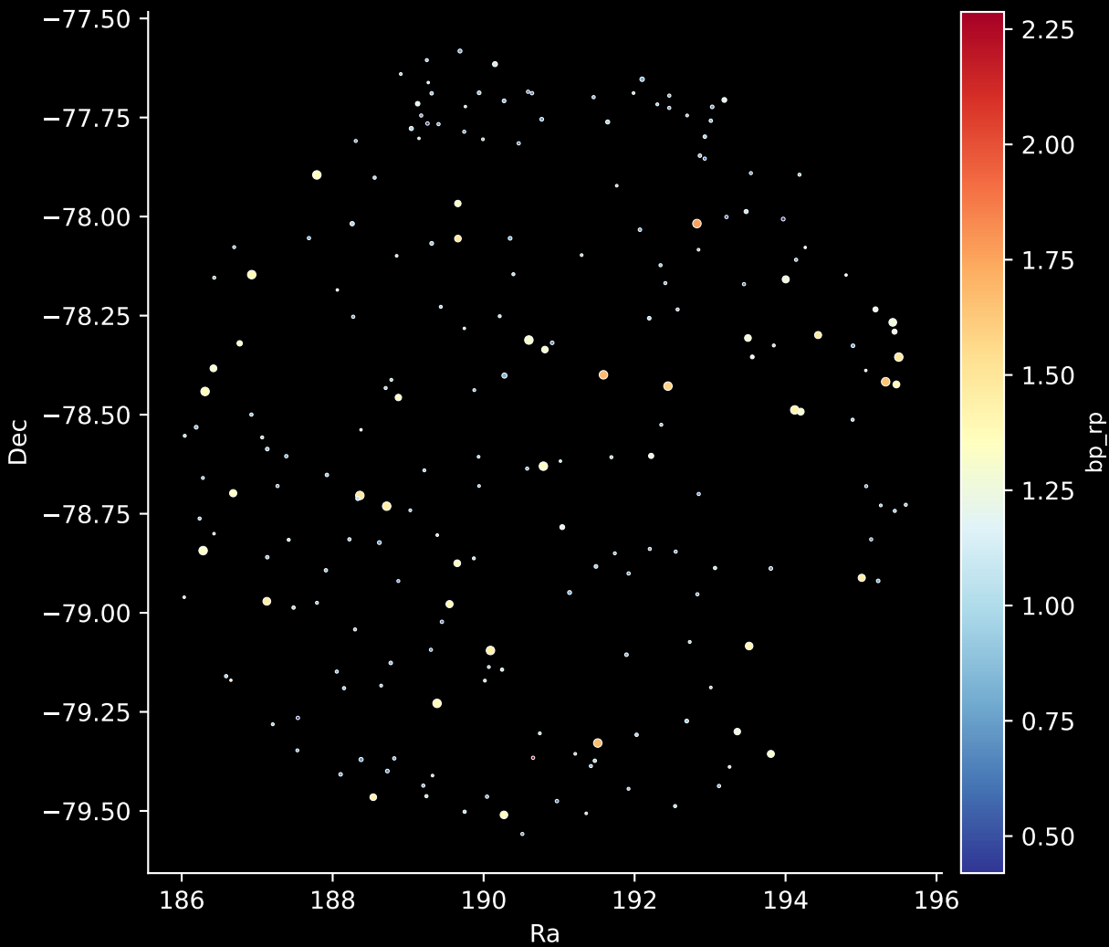
GALAH DR4 Field: [7238] Stars: 209
