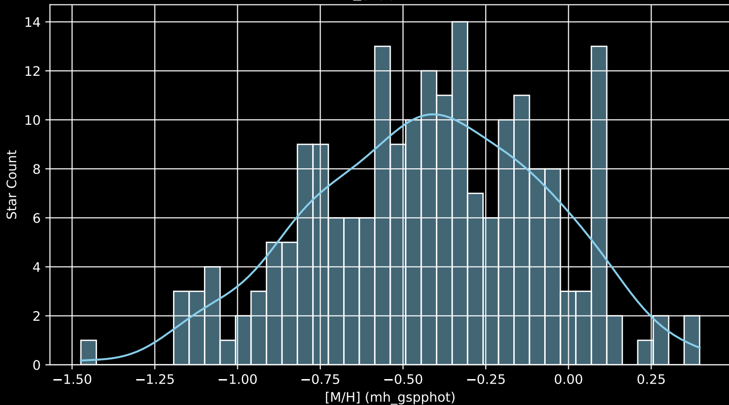
GALAH DR4 Field: [7238] [M/H] (mh_gspphot) (n= 208)
