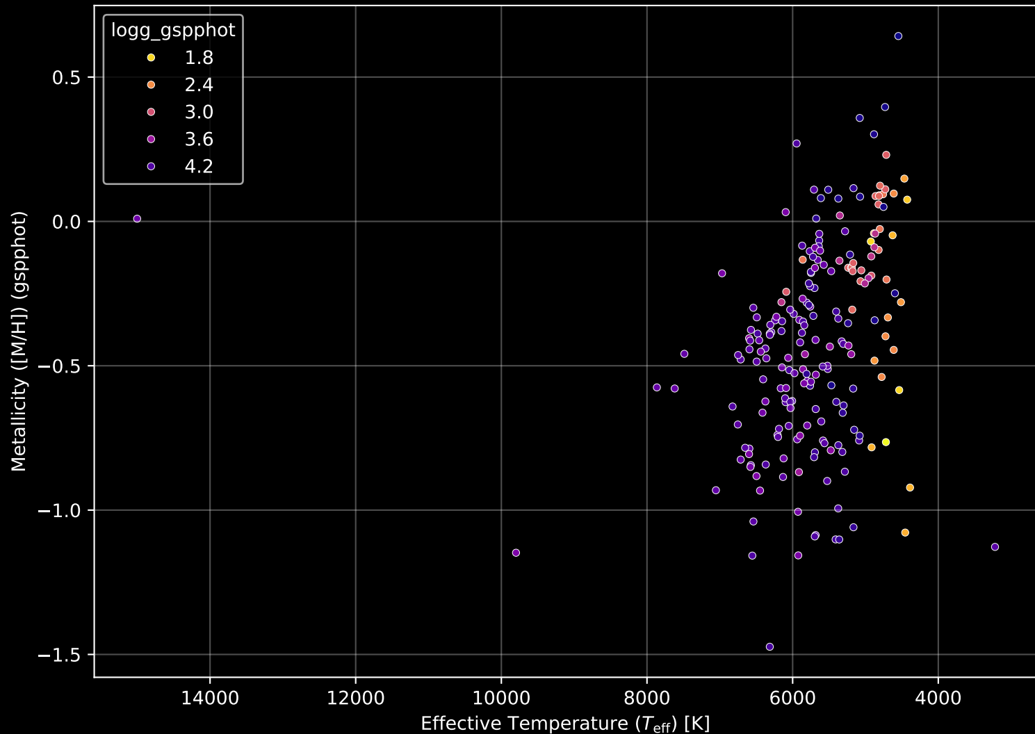
GALAH DR4 Field: [7238] Stellar Population Parameters (n= 209)
